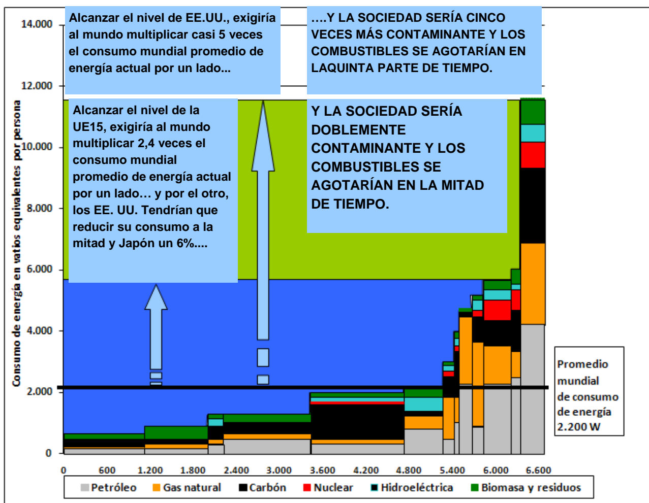
Figura 5: Consumo de energía en vatios equivalentes por persona.
