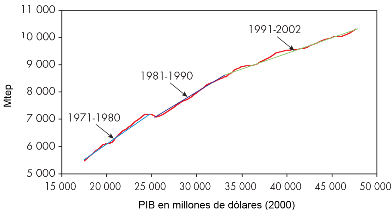
Figura 7: PIB y demanda de energía primaria mundial 1971 - 2002.
