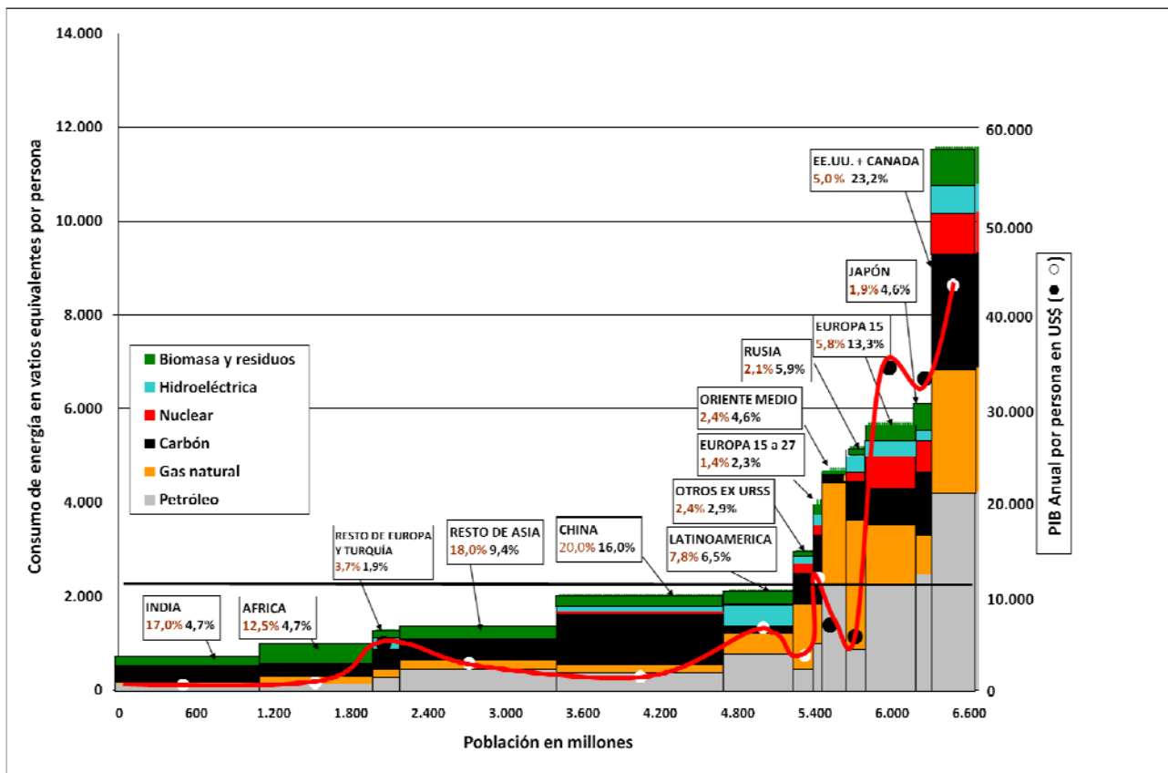
Figura 1: Consumo de energía en vatios equivalentes por persona y PIB per cápita anual, por zonas geográficas y fuentes energéticas primarias.
